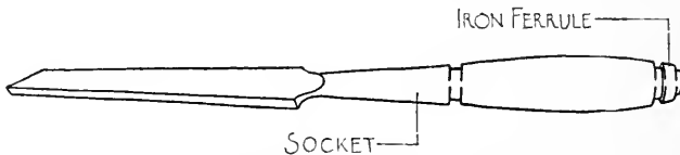
FIG. 48. MORTISE CHISEL.
